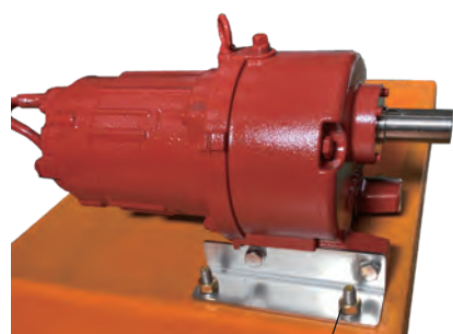
ナット(真中) M12 パネ座金(SUS) M12
